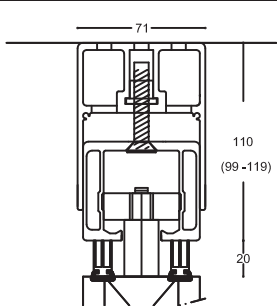
1. Säädettävä kiskosto suora
