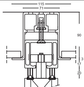
2. Säädettävä kiskosto alakattolistoin
