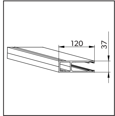
ohjauskisko 120 x 37 mm
