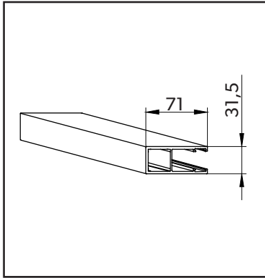
ohjauskisko 71 x 31,5 mm
