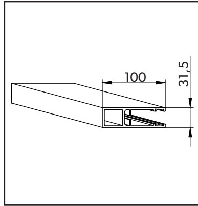
ohjauskisko 100 x 31,5 mm
